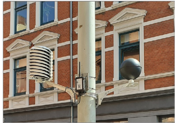
Abb. 79: Beispiel einer Klimamessstation mit Lufttemperatur-/Feuchte-Sensorik in Strahlungsschutzgehäuse (links) und Globe-Temperaturmessung (rechts).
