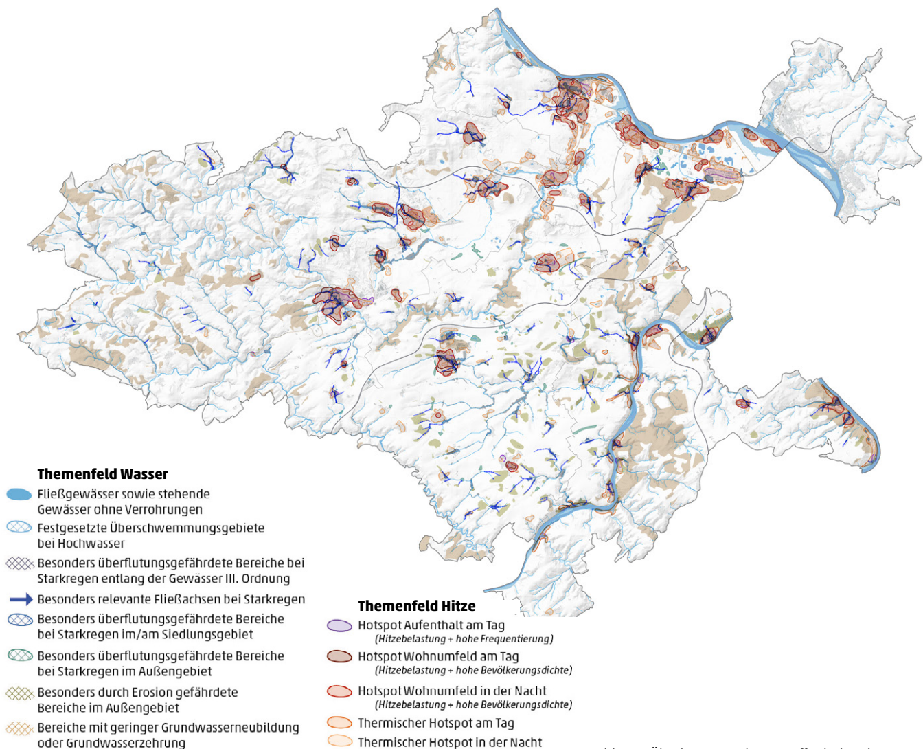
Abb. 34: Überlagerung der Betroffenheiten in MYK
